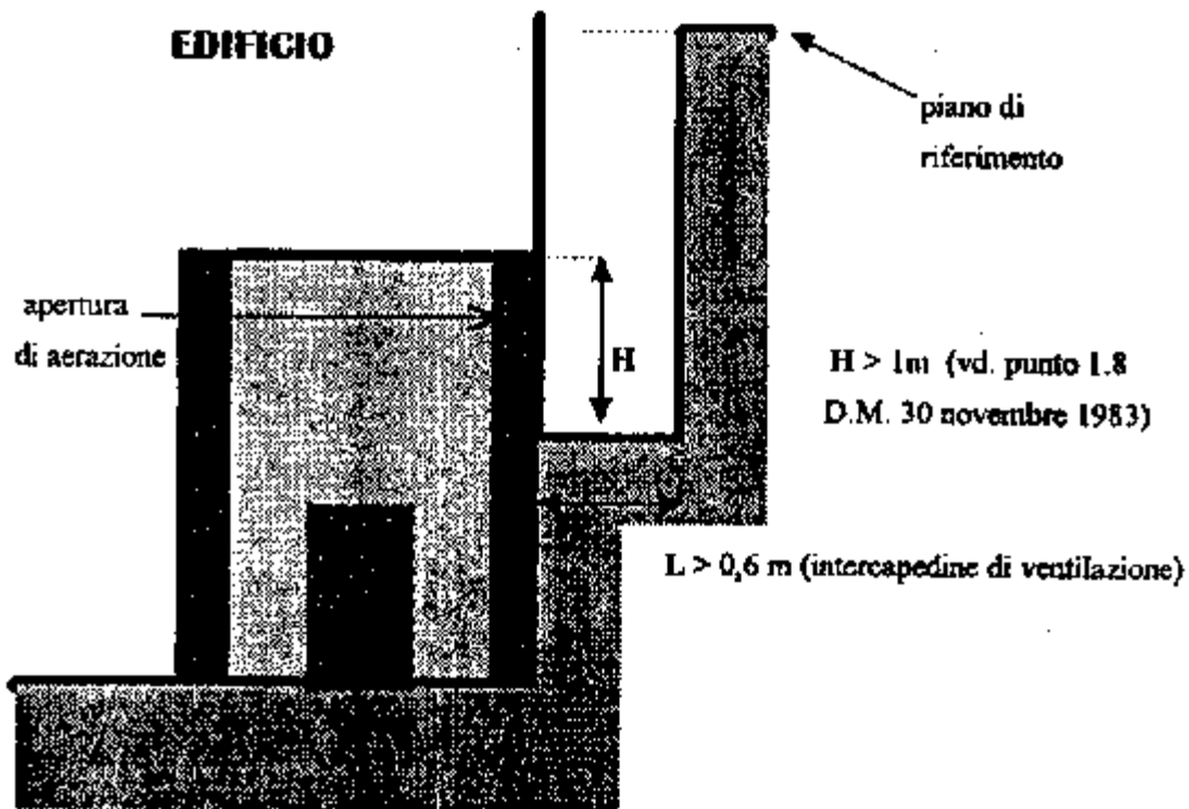
Tavola 2a - locale interrato
