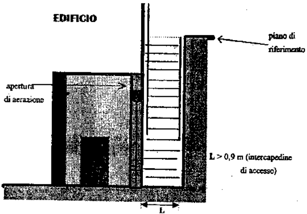
Tavola 2a - locale interrato
